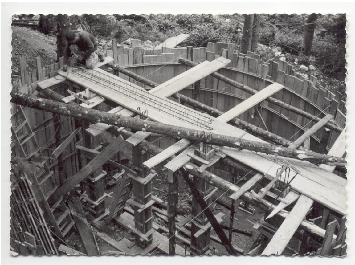
Armatura della trave di collegamento diametrale
